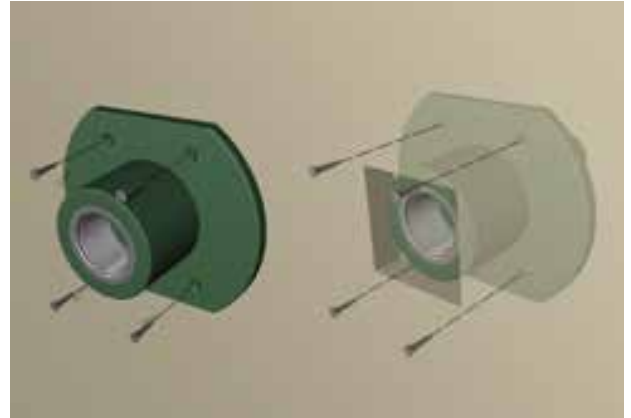
Paso 3: Fijar la Cupla Dry Fix al tabique con los tornillos.
