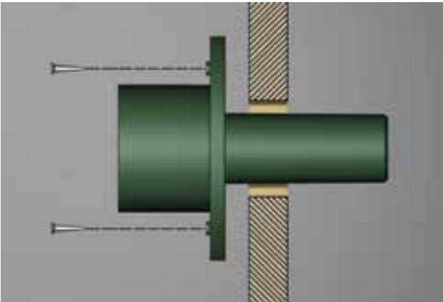
Paso 2 A: Según el proyecto, verificar si se quiere colocar la cupla por delante o por detrás del tabique. Realizar las perforaciones correspondientes en la solapa de la cupla y limpiar las rebabas.
