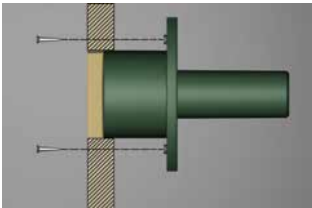
Paso 2 B: En caso de que quiera colocar la cupla por delante.
