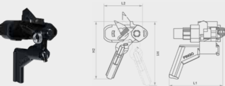
DIMENSÕES (MM)
