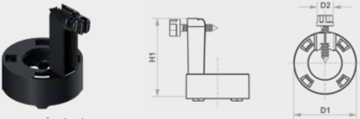
DIMENSÕES (MM)
