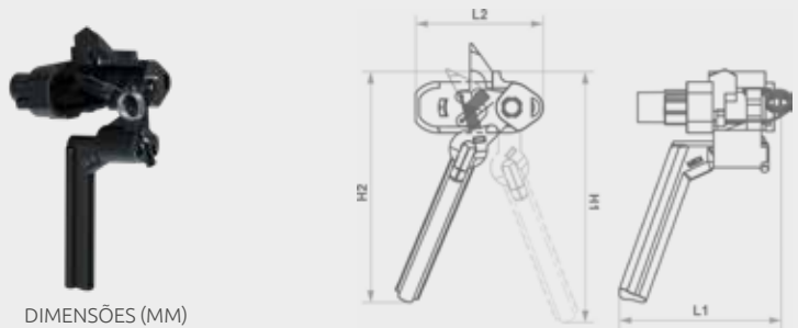
DIMENSÕES (MM)
